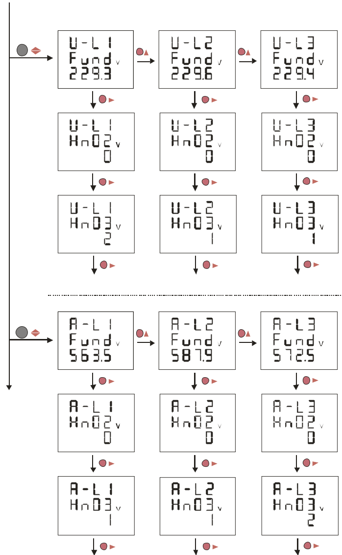
Figura 61 . Visualización de Descomposición Armónica en Tensión y Corriente
